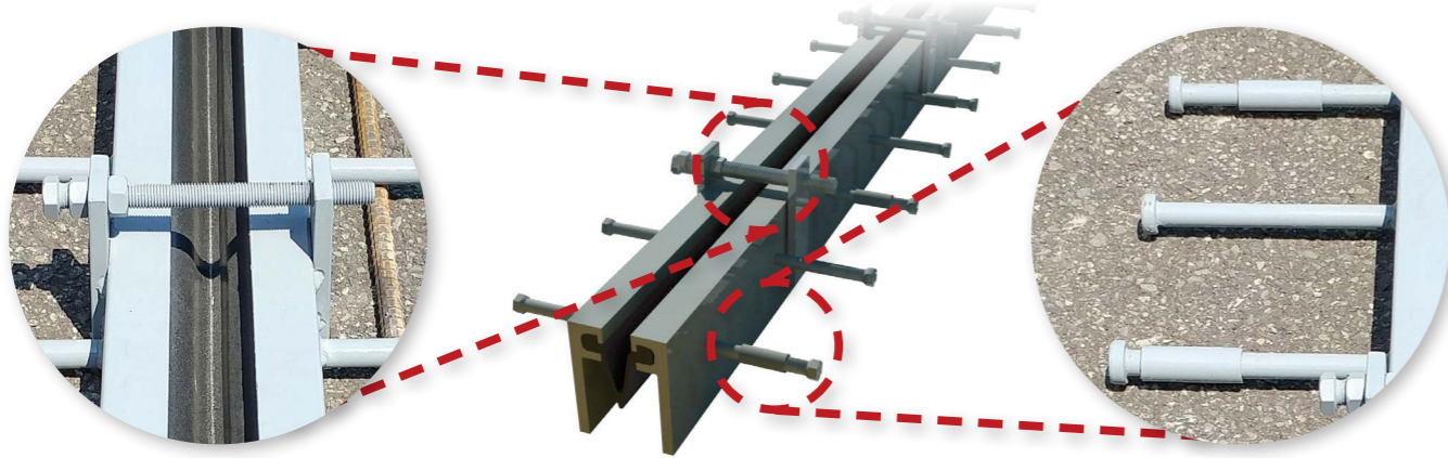
프리세팅 장치로 현장에서 정밀한 유간 조정 가능
