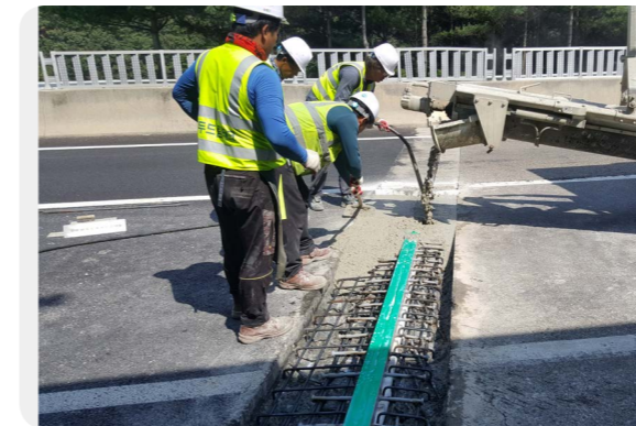
무수축 몰탈 타설
