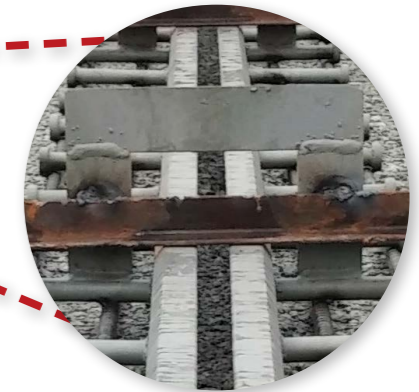
수평 유지를 위한 용접 고정
