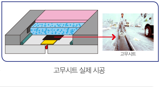
일체 신축으로 괴리현상 없음
