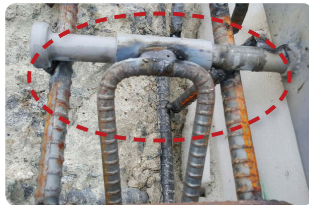
프리세팅 덕트로 인해 유간 조정 시 뒤틀림이 발생하지 않음
